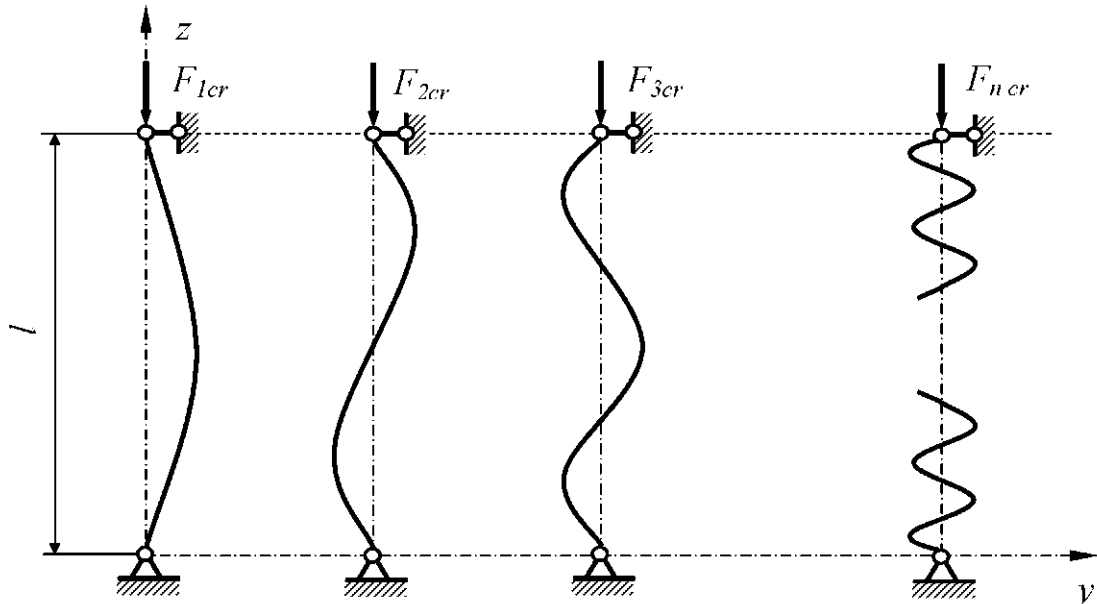
Рис. 2.3. Формы потери устойчивости сжатого стержня
