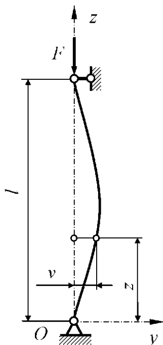
Рис. 2.2. Задача Эйлера
